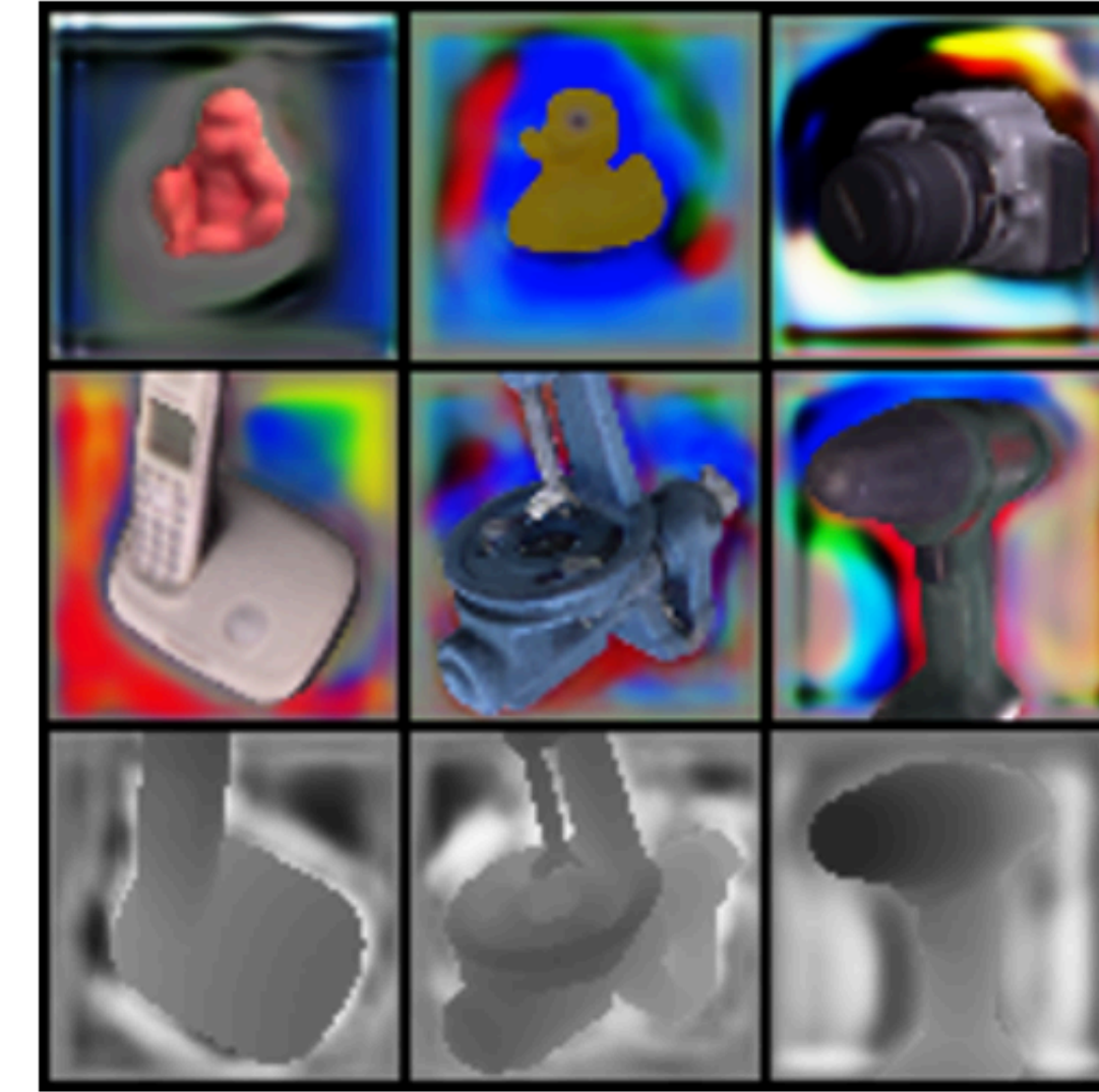
DeceptionNet
